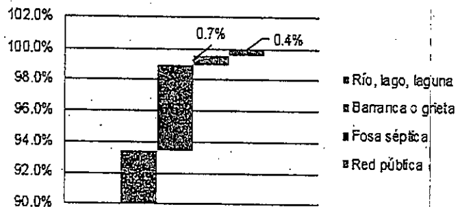
Vía de disposición del drenaje
